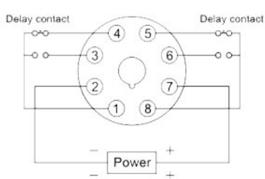
DH48S-S-2Z, DH48S-2Z
