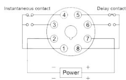
DH48S-2ZH
