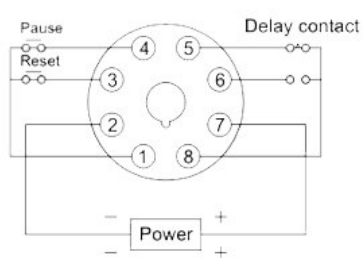
DH48S-S, DH48S-1Z
